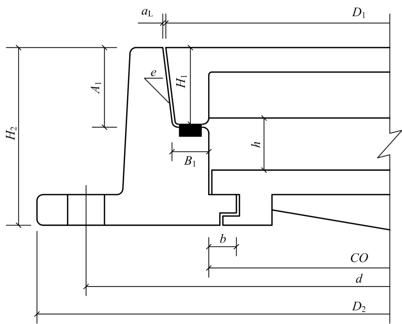
图 1 检查井盖座示意
