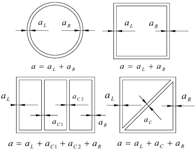
图2 检查井盖总间隙
