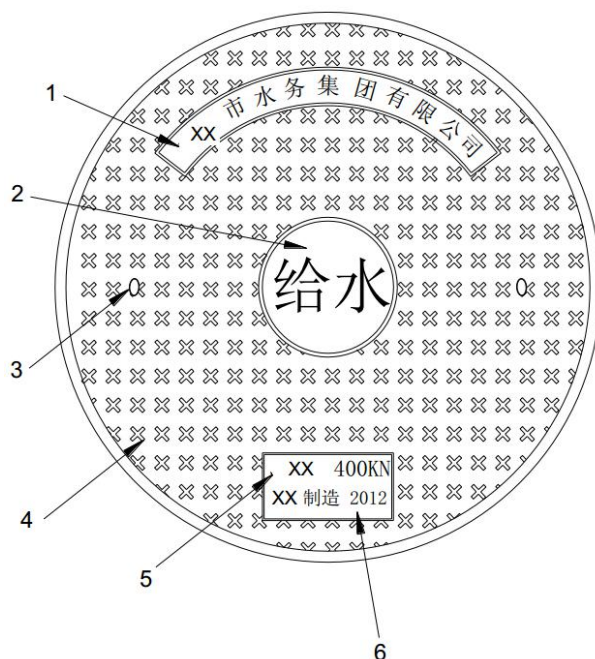
附图 1 检查井盖外观及标识示例
