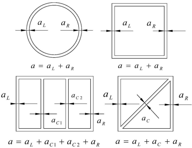
图 3.2.2 检查井盖间隙尺寸示意图
