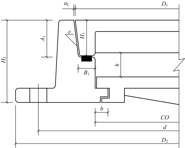
图 3.2.1 检查井盖结构尺寸示意图
