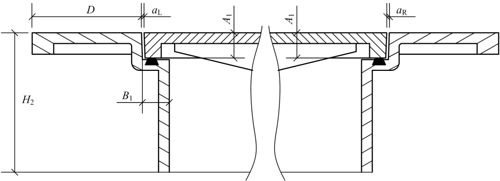
图 3.2.3 防沉降检查井盖结构尺寸示意图
