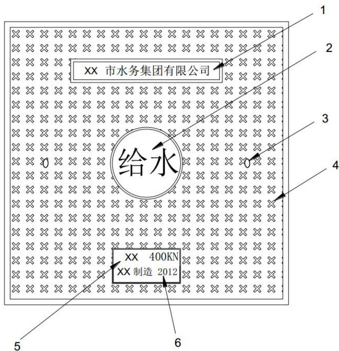
球墨铸铁或复合材料圆形检查井盖外观及标识示例图
