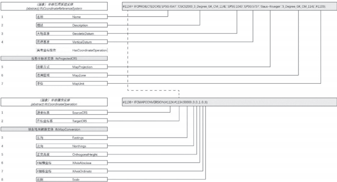
图6 坐标实体存储分类信息的方式
