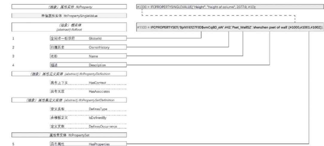
图2 属性集实体存储方式
