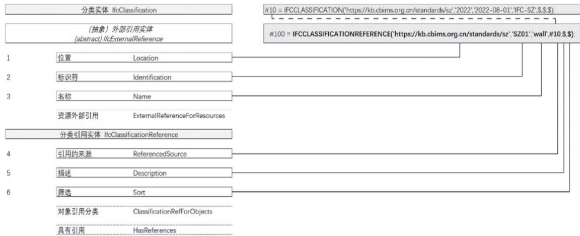
图4 分类引用实体存储方式
