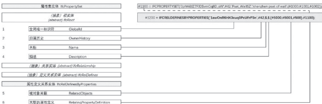
图3 属性定义关系实体存储方式
