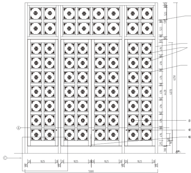
图 5.4 铜门设计图
