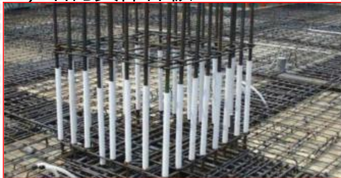
楼板绑扎样板
